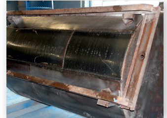
Uusi pohjalevy hitsataan kuten uuden säiliön sauma
